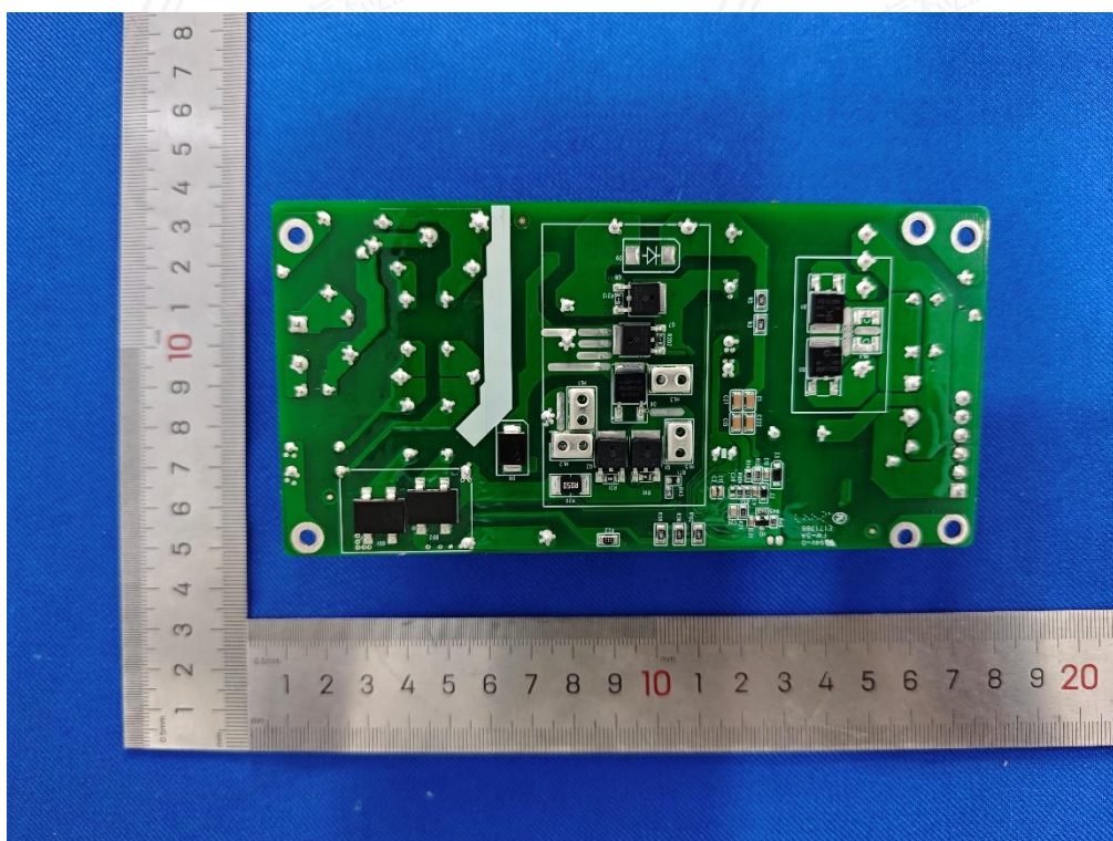
照片 12 内部电源反面
