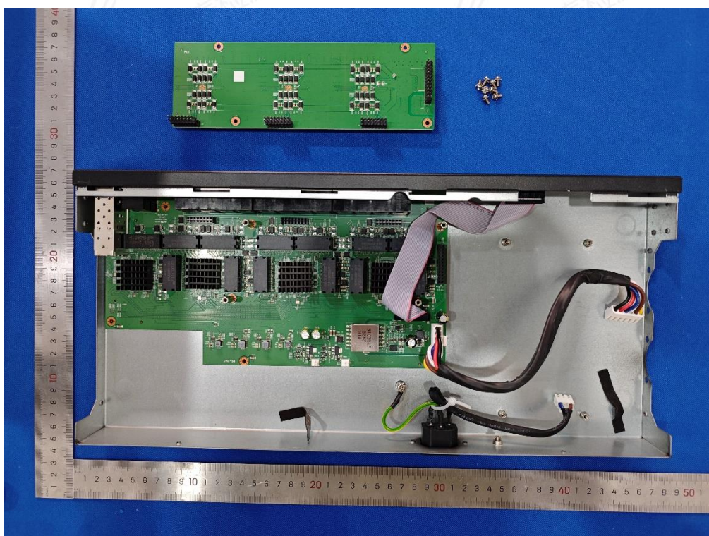
照片 14 内部视图
