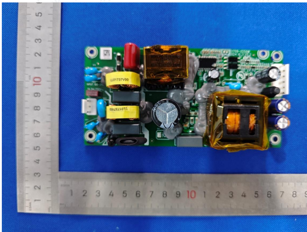
照片 11 内部电源正面
